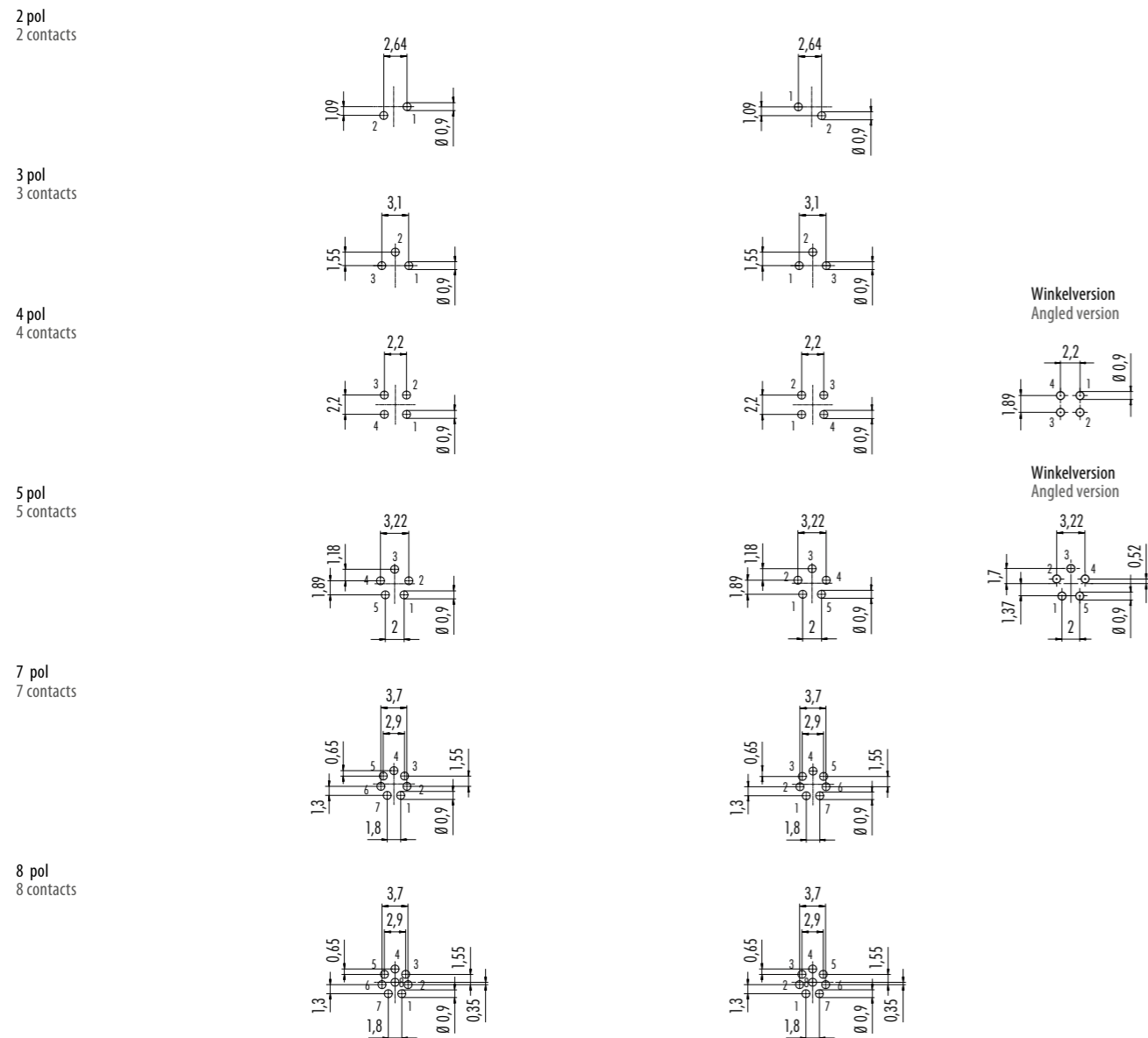
Bohrbilder Stifteinsatz (Leiterplatte) Drilling schemes male insert (PCB)
